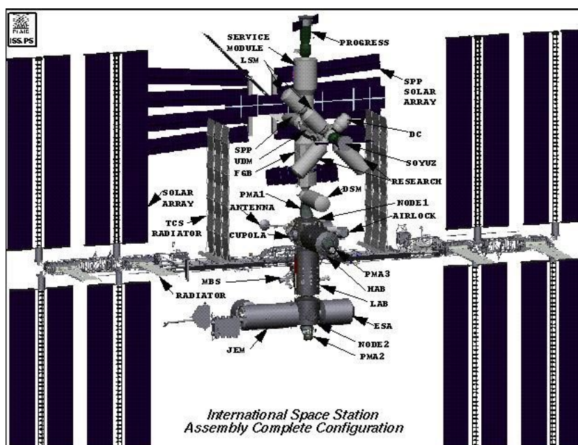
МКС
