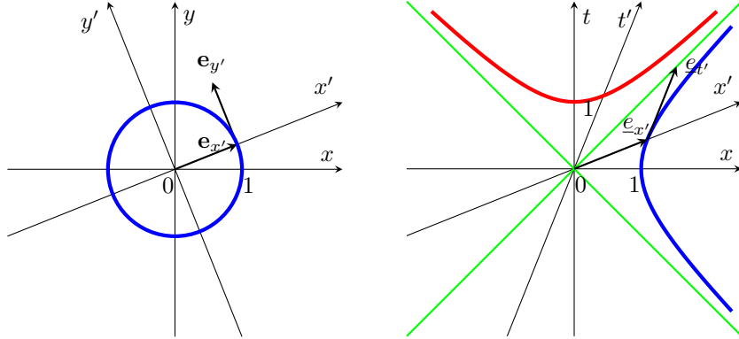
Дифференцирование базисного вектора \underline{e}_{x'}/\underline{e}_{x'} по естественному параметру вдоль окружности/гиперболы даёт второй базисный вектор.
